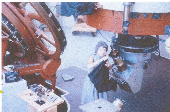
Vera Rubin installant son spectromètre au 72-in telescope du Lowell Observatory en 1965 (@ The Carnegie Institution for Science – Rubin Collection).
