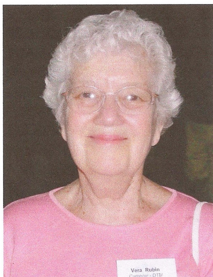
Vera Rubin vers 2010 (@ Michael A. Stecker).
